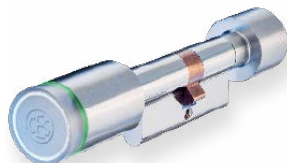
Dubbele knopcilinder voor overbrengingsloten F815DK-X-GS
